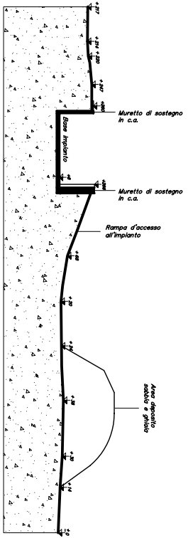
SEZIONE C-C
